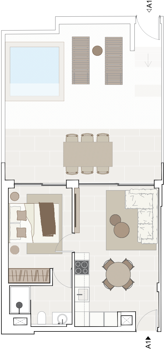
Vivienda A1. E = 1/30
